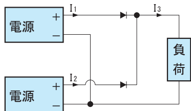
図 4.2 冗長運転例
