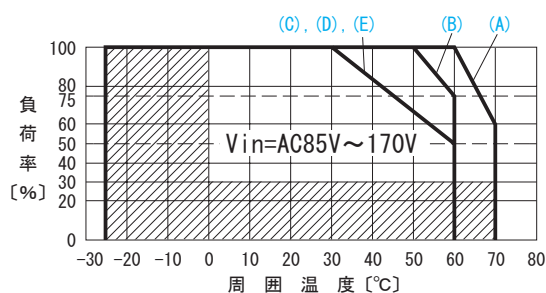
図 5.13 動作周囲温度によるディレーティング特性 (Vin = AC85 ~ 170V)
