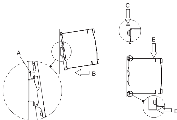
図 5.2 取付方法
