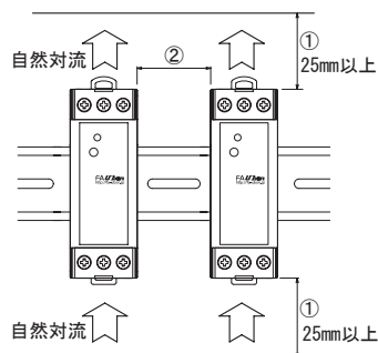
図 5.3 取付間隔
