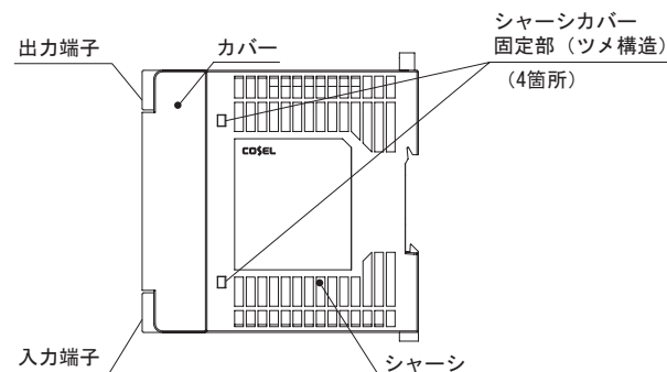
図 5.24 シャーシカバー取り外し説明図
