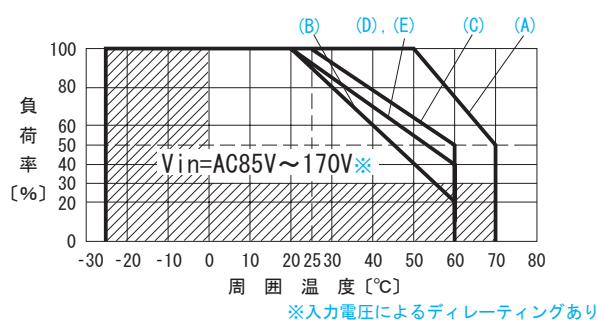
図 5.17 動作周囲温度によるディレーティング特性 (Vin = AC85 ~ 170V)
