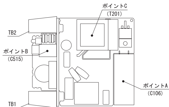
図 5.21 温度測定ポイント（強制通風時）
