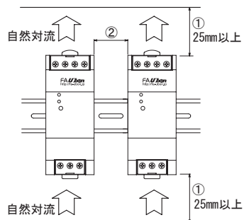
図 5.4 取付間隔
