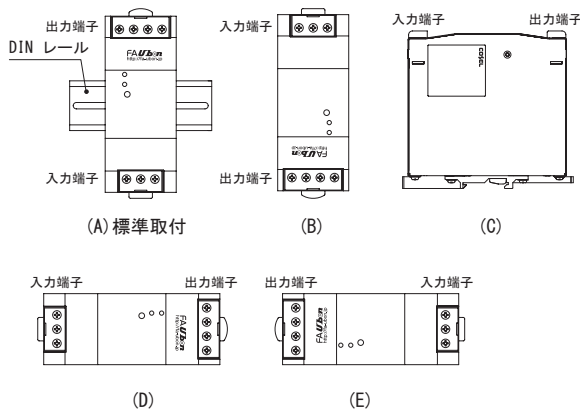
図 5.1 取付方向
