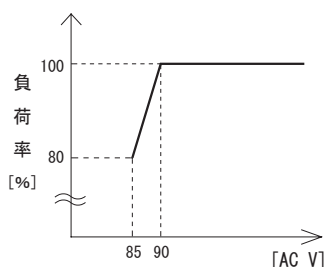
図 5.5 入力電圧によるディレーティング
