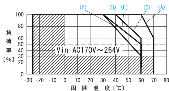
図 5.18 動作周囲温度によるディレーティング特性 (Vin = AC170 ~ 264V)
