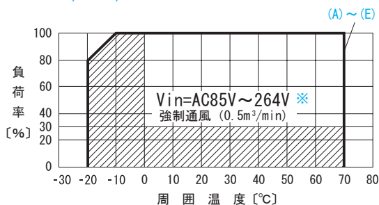
図 5.20 動作周囲温度によるディレーティング特性 (Vin = AC85 ~ 264V)
