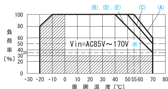
図 5.9 動作周囲温度によるディレーティング特性 (Vin = AC85 ~ 170V)
